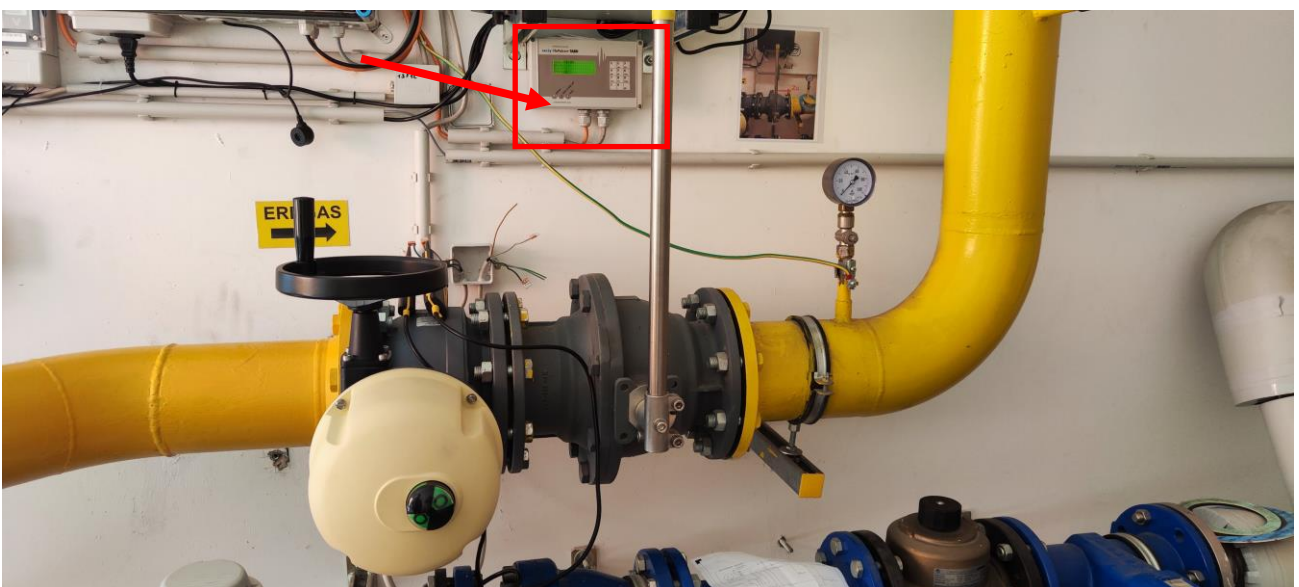
Zentrale Bedieneinheit TABD
